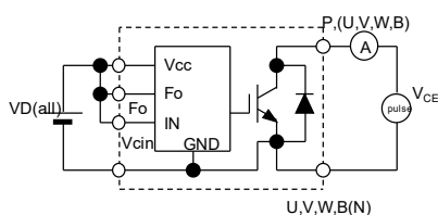
Fig.5 I_{CES} Test
