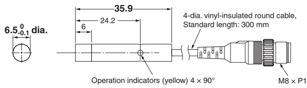
E2E-C06N04-CJ-□□
