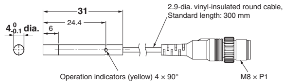
E2E-S04N02-CJ-□□
