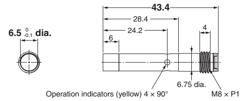
E2E-C06N04-MC-□□
