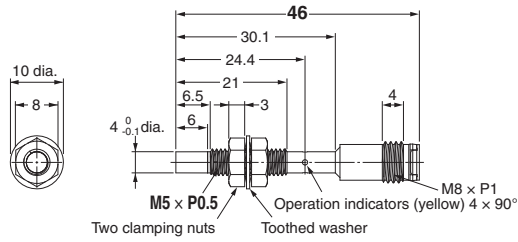
E2E-S05N03-MC-□□
