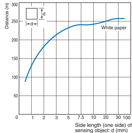
E3Z-L□1(L□6)
