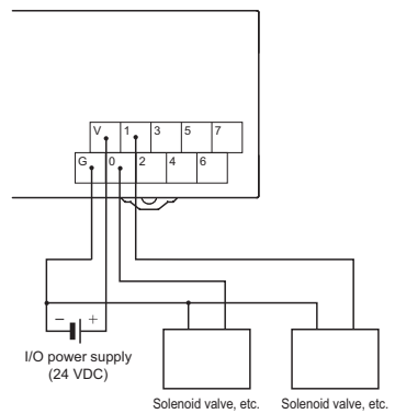
XWT-OD16-1 (PNP)
