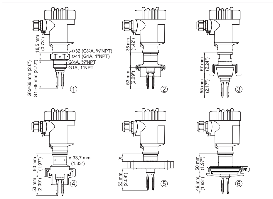
Fig. 18: VEGASWING 61
