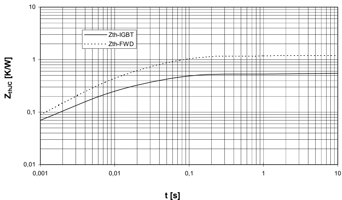
Transienter Wärmewiderstand Wechsele. Transient thermal impedance Inverter
