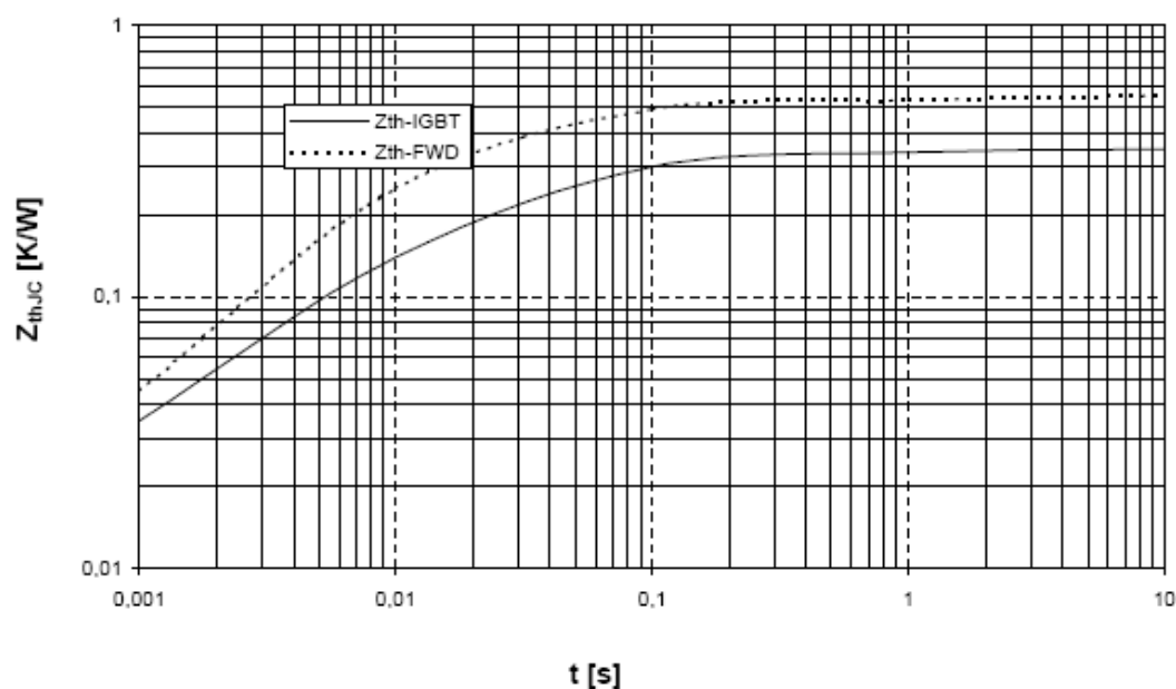
Transienter Wärmewiderstand Wechslr. Transient thermal impedance Inverter
