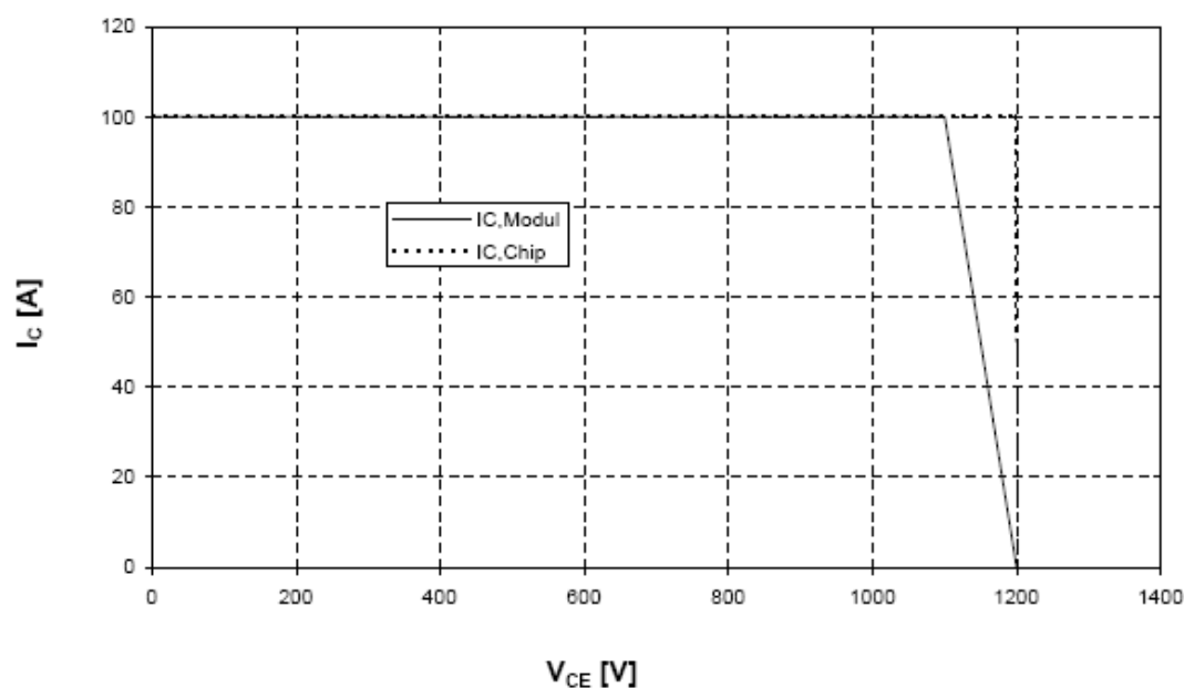
Sicherer Arbeitsbereich Wechslr. (RBSOA)
