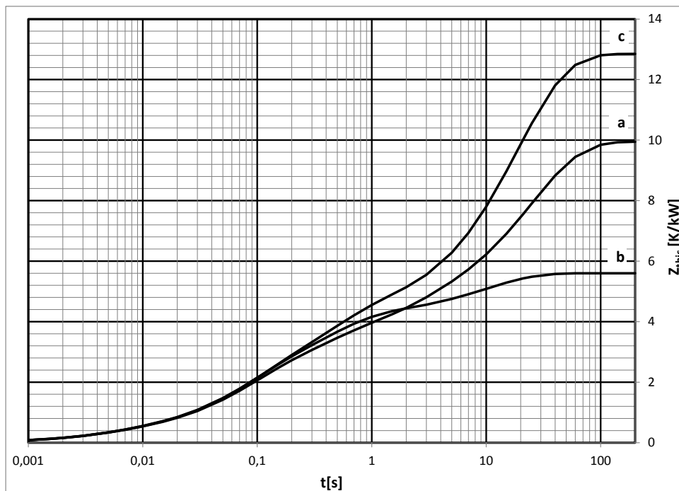
Transienter innerer Wärmewiderstand für DC / Transient thermal impedance Z_{thJC} = f(t) for DC
