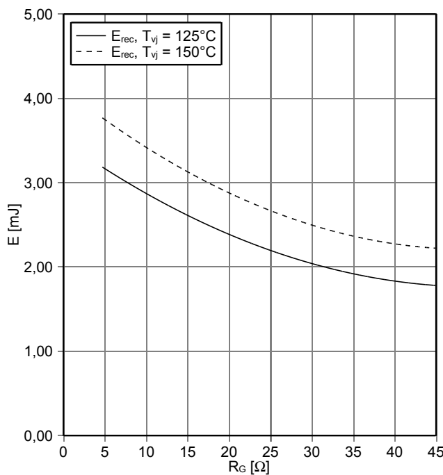
Schaltverluste Diode-Chopper (typisch) switching losses Diode-Chopper (typical)
