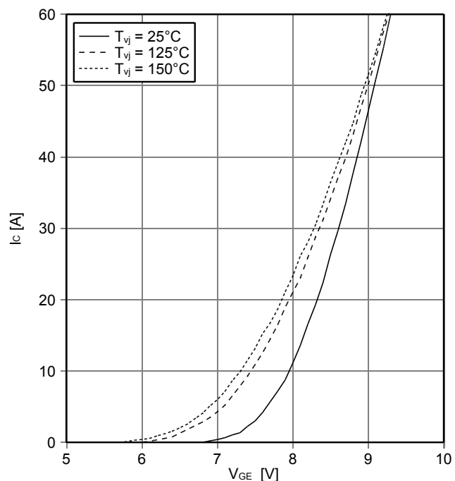
Übertragungscharakteristik IGBT-Chopper (typisch) transfer characteristic IGBT-Chopper (typical) I_C = f(V_{GE}) V_{CE} = 20\text{ V}
