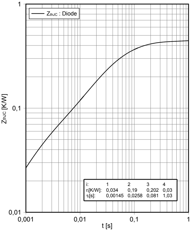
Transienter Wärmewiderstand Diode, Wechselrichter transient thermal impedance Diode, Inverter Z_{thJC} = f(t)
