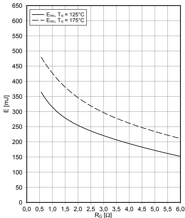
Schaltverluste Diode, Wechselrichter (typisch) switching losses Diode, Inverter (typical) E_{rec} = f(R_G)
