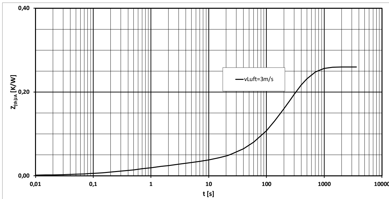
Transienter Wärmewiderstand je Zweig / Transient thermal impedance per arm Z_{thJA} = f(t)
